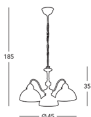
■ 731.83.126 Luster / chandelier ☐ 3 lp., E27, 75 W / LED E27
