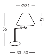
264.71.7 Tischleuchte / table lamp Messing / brass 1 lp., E27, 60 W / LED E27
