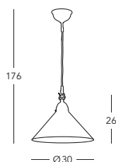
731.30.10 Hängeleuchte / hanging lamp 1 lp., E27, 75 W / LED E27
