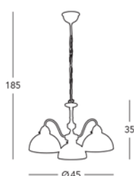
■ 731.83.150 Luster / chandelier ☐ 3 lp., E27, 75W / LED E27
