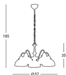
■ 731.85.170 Luster / chandelier □ 5 lp., E27, 75W / LED E27
