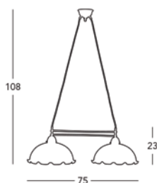
731.82.161 Balken / chandelier 2 l.p., E27, 75W/LED E27
