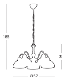
■ 731.85.122 Luster / chandelier ☐ 5 lp., E27, 75 W / LED E27
