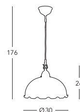
731.30.74 Hängeleuchte / hanging lamp 1 lp., E27, 75 W / LED E27
