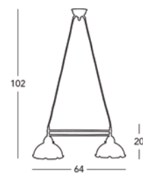
731.82.160 Balken / chandelier 2 l.p., E27, 75W/LED E27
