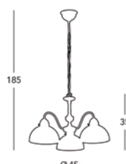
■ 731.83.16 Luster / chandelier □ 3 lp., E27, 75 W / LED E27
