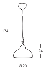
■ 731.30.103 Hängeleuchte / hanging lamp ☐ 1 lp., E27, 75 W / LED E27
